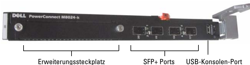
Abbildung 1-1. Vorderseite des PowerConnect M8024-k
